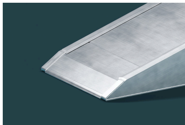
Lower end detail - Van
